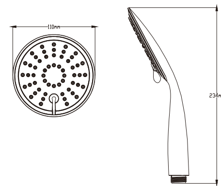
Maßzeichnungen
